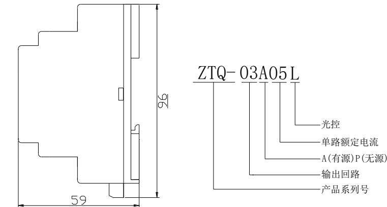
图 1-3（产品侧面尺寸）
