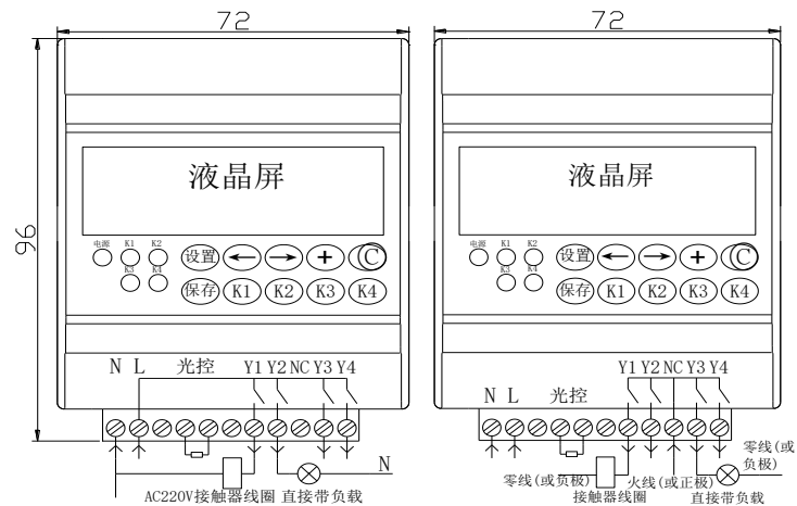
图 1-1（有源款尺寸以及电气接线参考）
